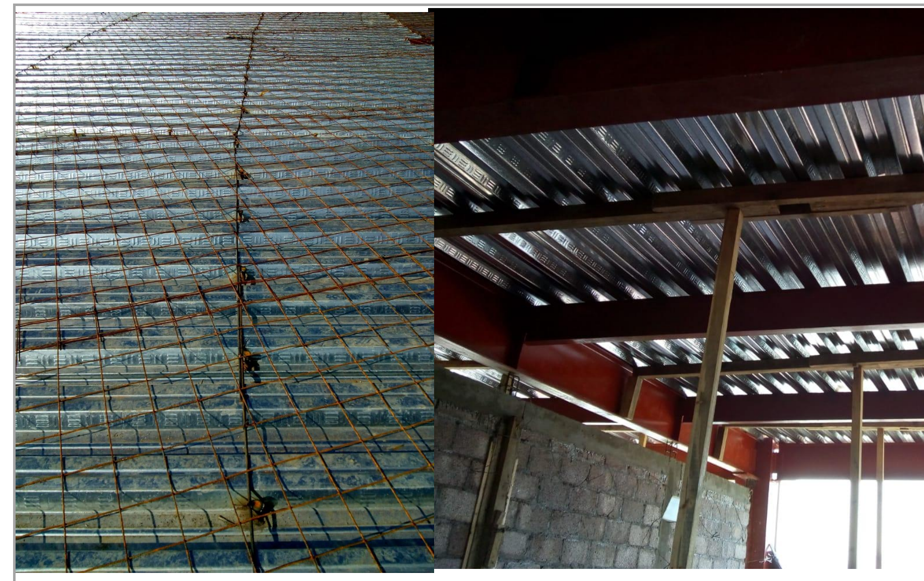
F2: PREPARACIÓN DE LOSACERO PARA COLADO DE CONCRETO.
