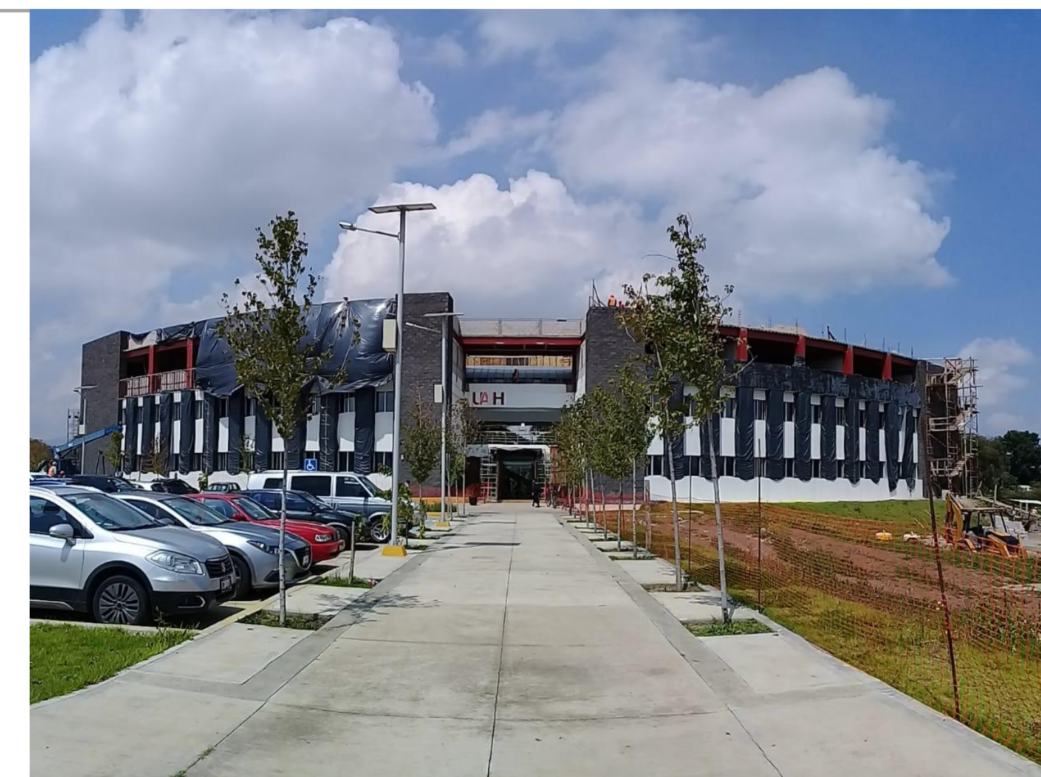
F5: VISTA DESDE FACHADA PRINCIPAL DONDE SE OBSERVA EL AVANCE DE LOS TRABAJOS PARA CONSTRUCCIÓN DEL 3ER PISO DE EDIFICIO DE AULAS EXISTENTE
