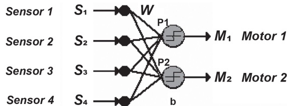
Figura 2. Red neuronal para la inclinación del seguidor.
