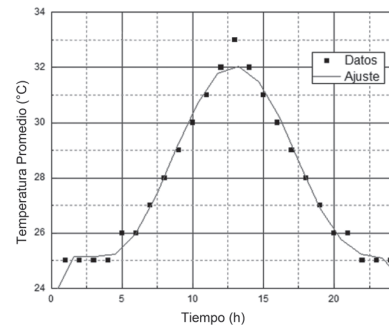
Figura 4. Respuesta del sistema mostrando el tiempo (h) versus temperatura.
