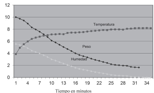
Figura 7. Determinación de la pérdida de peso y humedad en la flor de jamaica.
