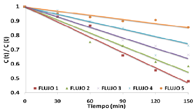
Figura 1. Variación de la concentración normalizada de plata a diferentes velocidades lineales de flujo cuando se aplica un potencial de celda controlado de 0.8V sobre dos electrodos de acero inoxidable 304 durante 150 minutos.
