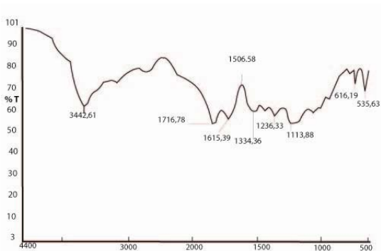
Fig. 2. Espectro infrarrojo obtenido en las fracciones de exclusión molecular, intercambio catiónico y aniónico.
