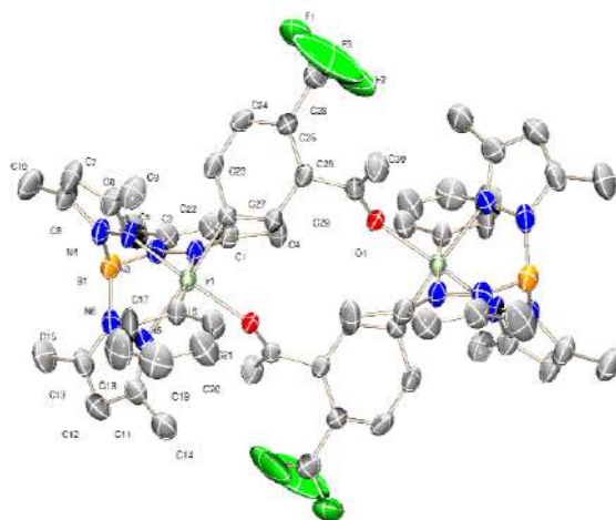
Figura 14. Perspectiva ORTEP de la estructura molecular del compuesto 5 grupo espacial P2_1/c con probabilidad de elipsoides 50%. (Se omiten los átomos de hidrógeno para la mejor visualización).
