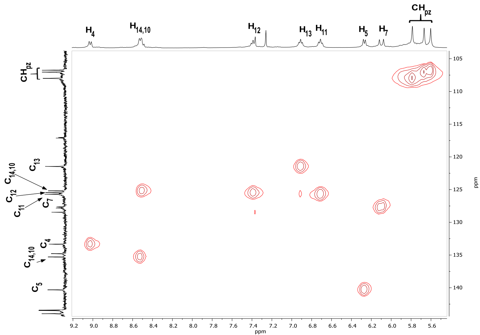
Figura 5. Ampliación del espectro HSQC en CDCl 3 para 4.
