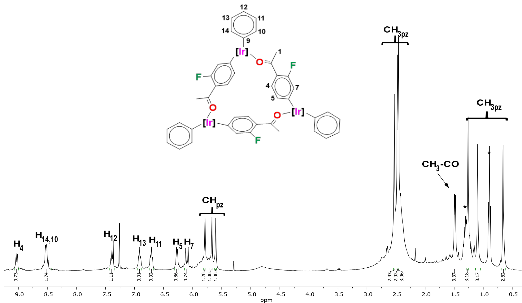
Figura 3. Espectro de RMN de ^1\text{H} para el complejo 4 a 400 MHz en \text{CDCl}_3 . *impurezas
