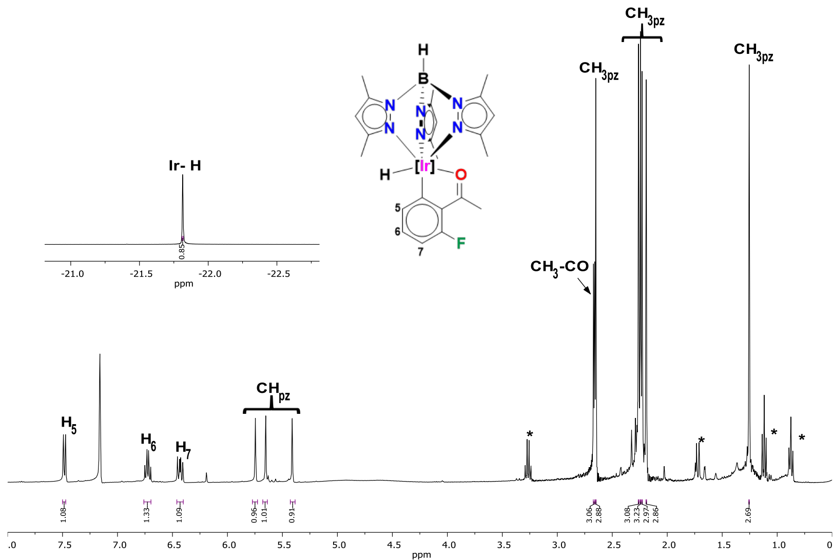
Figura 23. Espectro de RMN de ^1\text{H} para el complejo 8 a 400 MHz en \text{C}_6\text{D}_6 . *impurezas
