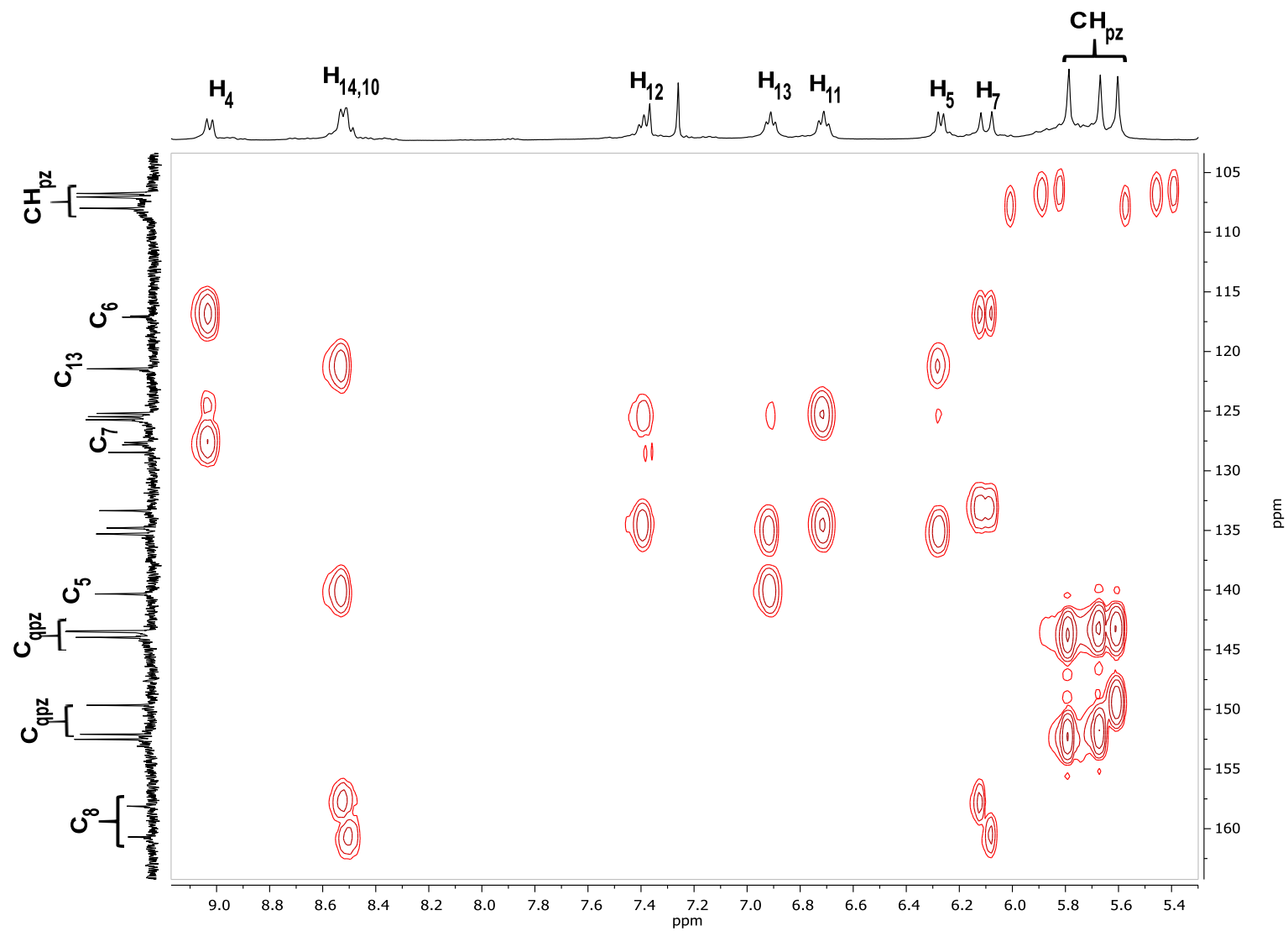
Figura 6. Ampliación del espectro HMBC en CDCl 3 para 4 .
