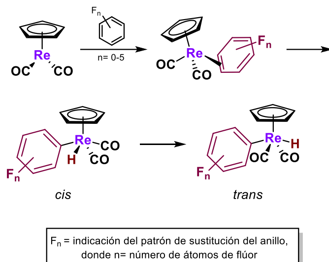
Esquema 12. Reactividad del complejo [\text{CpRe}(\text{CO})_2] con bencenos fluorados.
