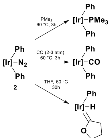
Esquema 4. Reactividad del complejo [Tp Me2 Ir(C 6 H 5 ) 2 (N 2 )].
