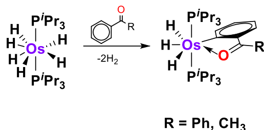
Esquema 8. Activación del enlace ortho -CH de acetofenona y benzofenona mediante el complejo [\text{OsH}_6(\text{P}^i\text{Pr}_3)_2] .
