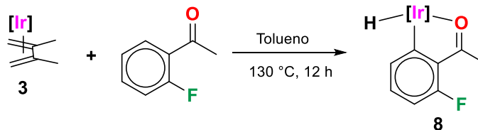
Esquema 17. Reactividad del complejo [\text{Tp}^{\text{Me}_2}\text{Ir}(\eta^4\text{-CH}_2=\text{C}(\text{Me})\text{C}(\text{Me})=\text{CH}_2)] con 1-(2-fluorofenil)etanona.
