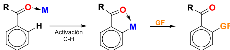
Esquema 6. Representación de la activación y funcionalización de enlaces C-H con grupos directores cetona (GF = grupo funcional).
