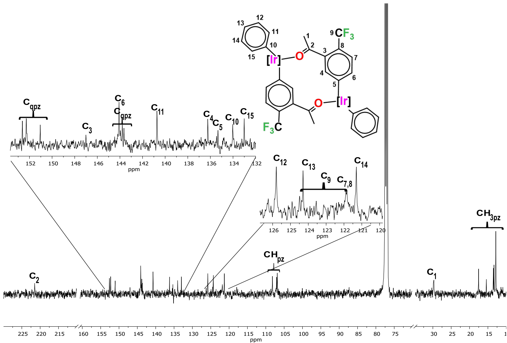
Figura 10. Espectro parcial de RMN de ^{13}\text{C} para el compuesto 5 a 100 MHz en \text{CDCl}_3 . *impurezas
