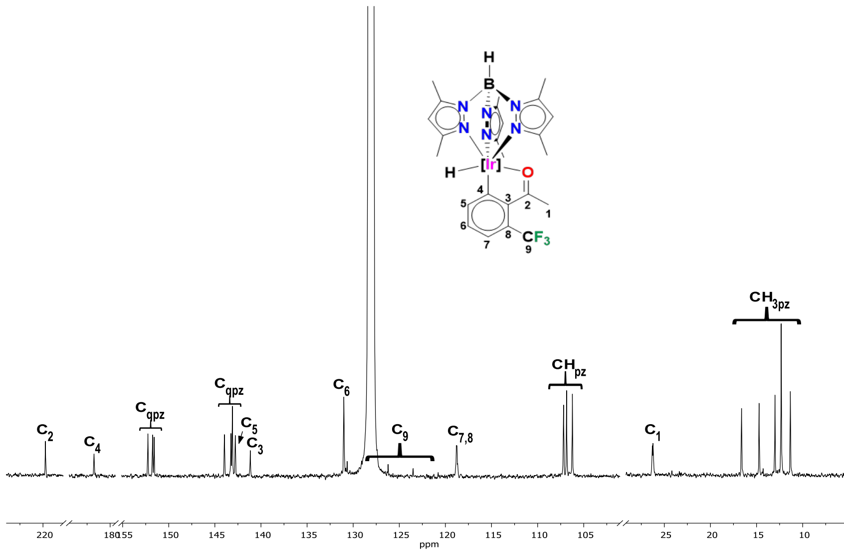
Figura 28. Espectro parcial de RMN de ^{13}\text{C} para el compuesto 9 a 100 MHz en \text{C}_6\text{D}_6
