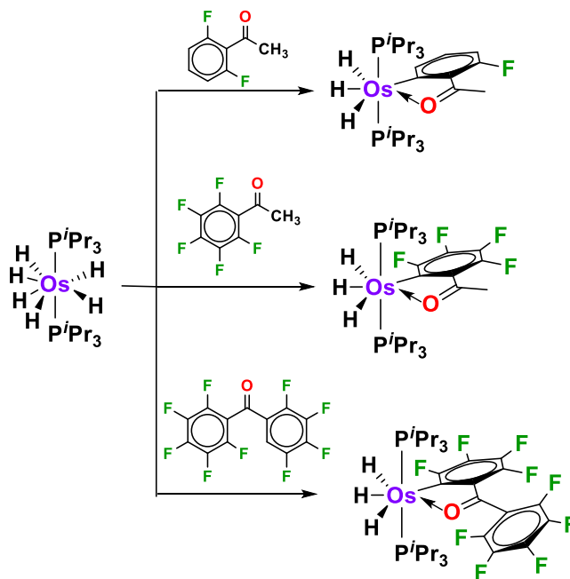
Esquema 9. Activación del enlace ortho -CF de cetonas fluoradas mediante el complejo [\text{OsH}_6(\text{P}^i\text{Pr}_3)_2] .
