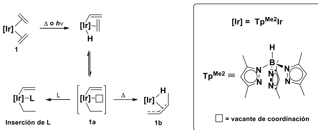
Esquema 1. Reactividad del complejo [\text{Tp}^{\text{Me}_2}\text{Ir}(\text{C}_2\text{H}_4)_2]
