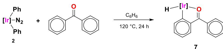
Esquema 16. Reactividad del complejo [\text{Tp}^{\text{Me}_2}\text{Ir}(\text{C}_6\text{H}_5)_2\text{N}_2] con benzofenona.
