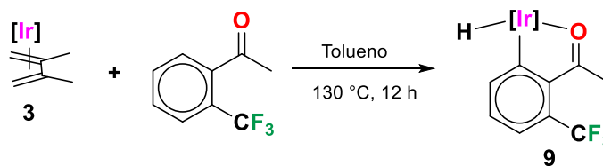
Esquema 18. Reactividad del complejo [\text{Tp}^{\text{Me}_2}\text{Ir}(\eta^4\text{-CH}_2=\text{C}(\text{Me})\text{C}(\text{Me})=\text{CH}_2)] con 2'-(trifluorometil)acetofenona.
