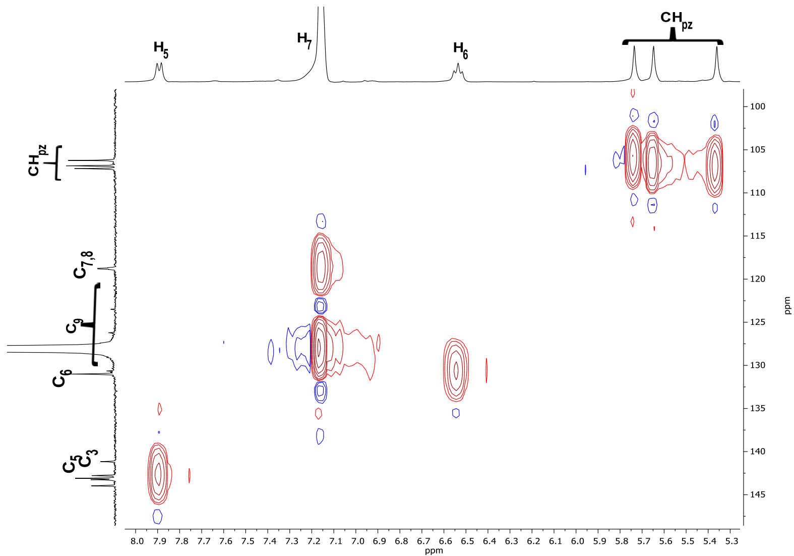
Figura 29. Ampliación del espectro HSQC en \text{C}_6\text{D}_6 para el compuesto 9.
