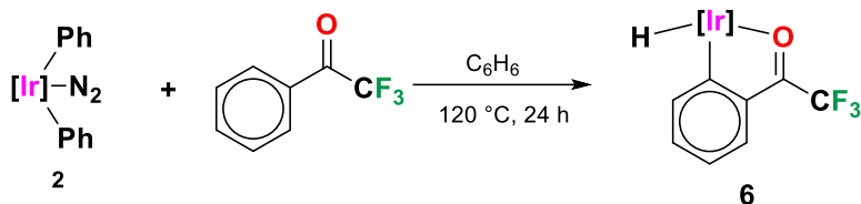
Esquema 15. Reactividad del complejo [\text{Tp}^{\text{Me}_2}\text{Ir}(\text{C}_6\text{H}_5)_2\text{N}_2] con la 2,2,2-trifluoroacetofenona.
