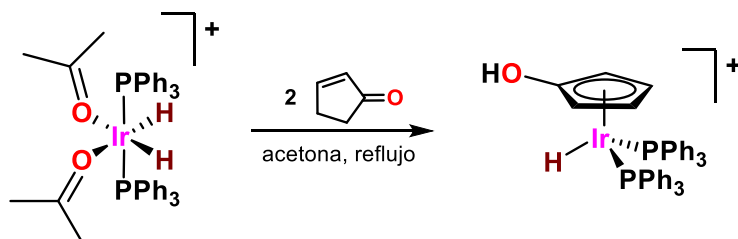
Esquema 11. Reactividad del ion complejo [\text{IrH}_2(\text{acetona})_2(\text{PPh}_3)_2]^+ con 2-ciclopentenona.
