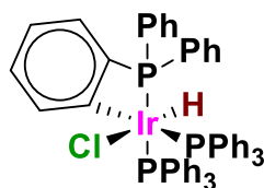
Figura 2. Primer ejemplo de metalaciclo de Ir.
