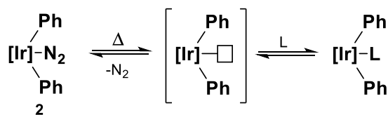
Esquema 3. Formación de la especie de 16 e - [Tp Me2 Ir(C 6 H 5 ) 2 ].
