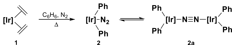
Esquema 2. Formación del complejo [\text{Tp}^{\text{Me}_2}\text{Ir}(\text{C}_6\text{H}_5)_2(\text{N}_2)]
