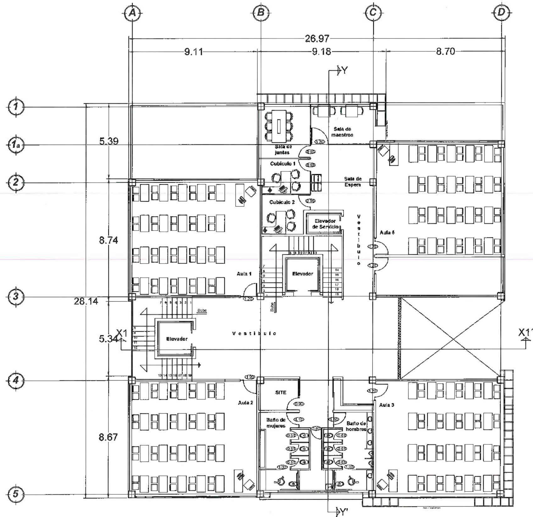
Planta 1er. Nivel
