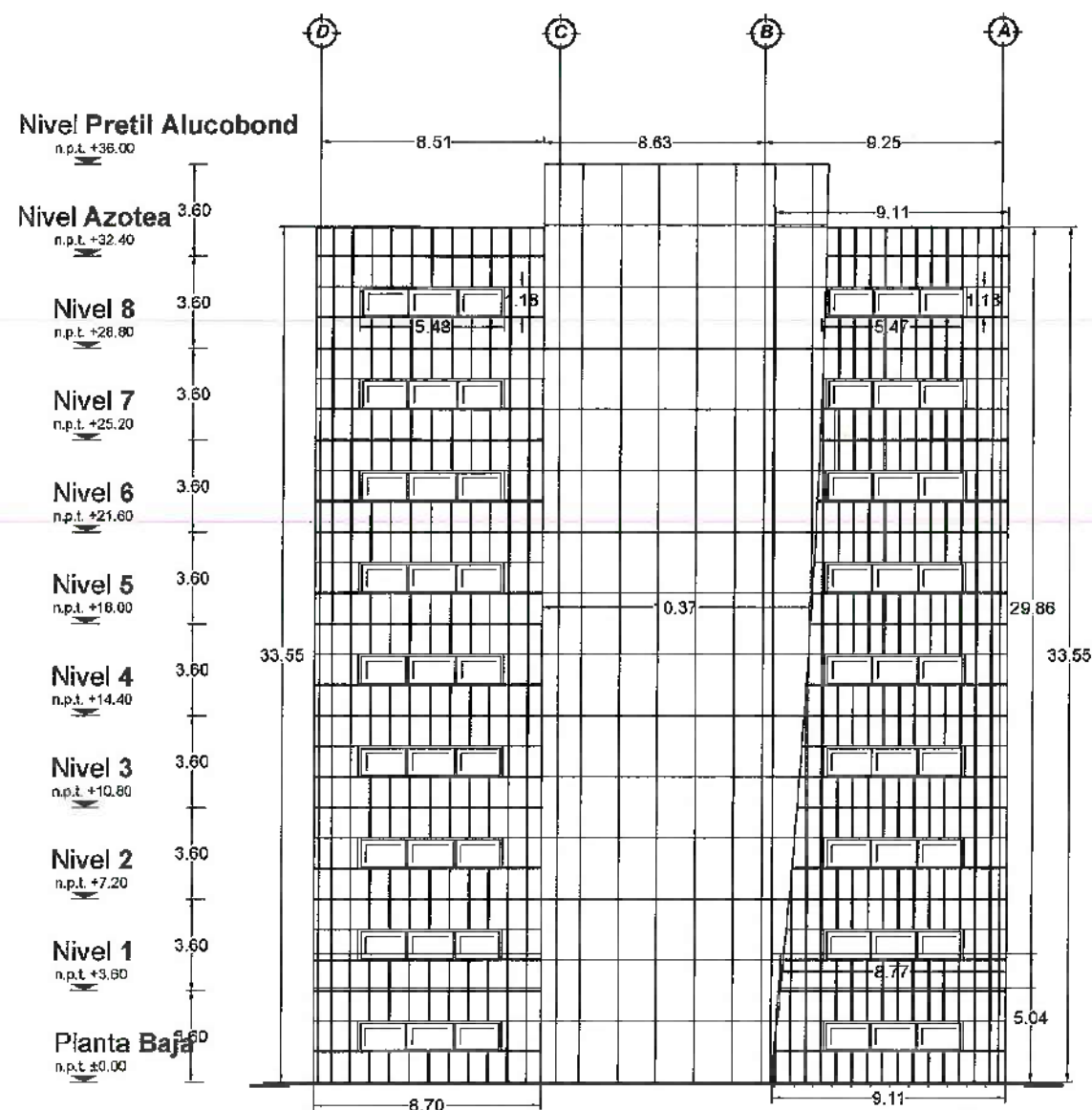
FACHADA PRINCIPAL ESTE
